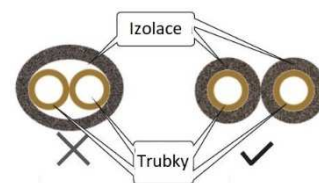
Obr. č. 38 – izolace potrubí chladiva
