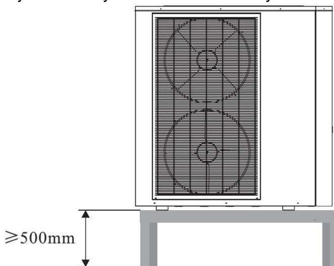
Obr. č. 23 – venkovní jednotka
