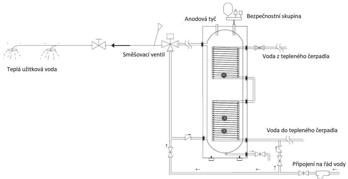
Obr. č. 17 – schéma zapojení t.u.v. 2
