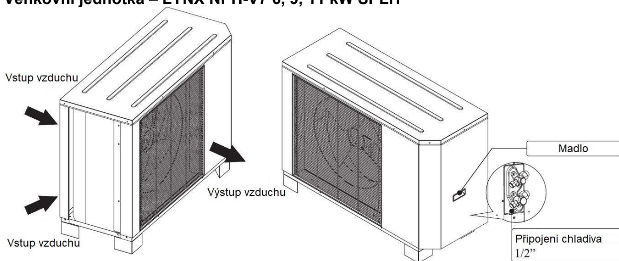
Obr. č. 5 – schéma venkovní jednotky LYNX NPH-V7 6, 9, 11 kW SPLIT
