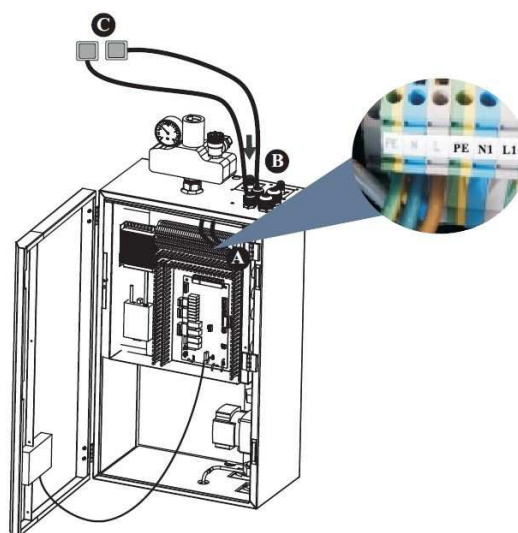
Obr. č. 32 – řídicí jednotka – napájení pomocného topení
