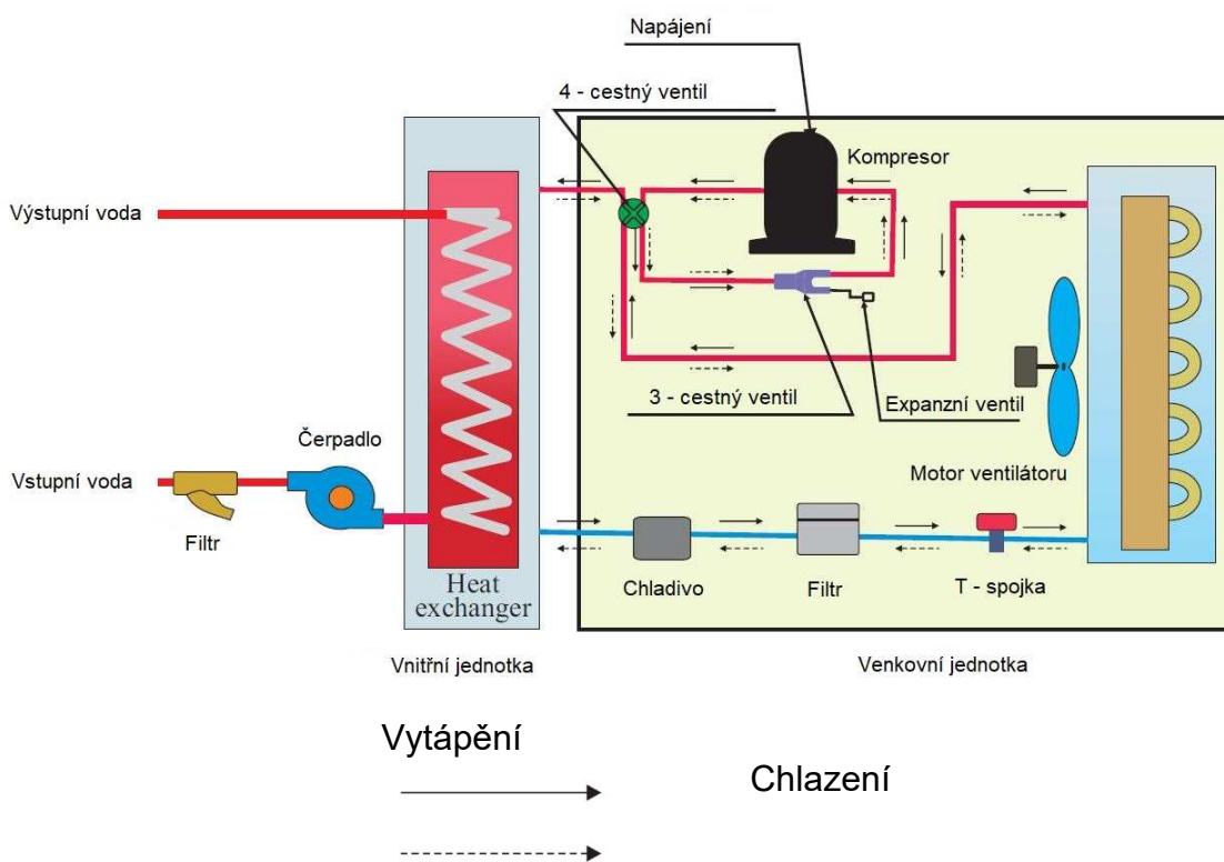
Obr. č. 2 – princip funkce zařízení
