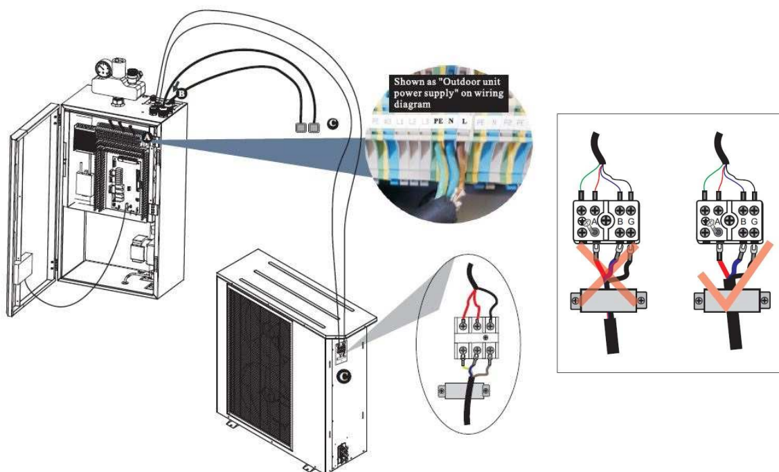
Obr. č. 34 – napájecí kabel mezi vnitřní a venkovní jednotkou
