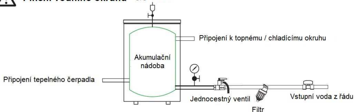
Obr. č. 1 – plnění vodního okruhu
