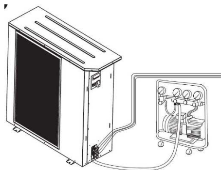
Obr. č. 43 – venkovní jednotka s vakuovou pumpou
