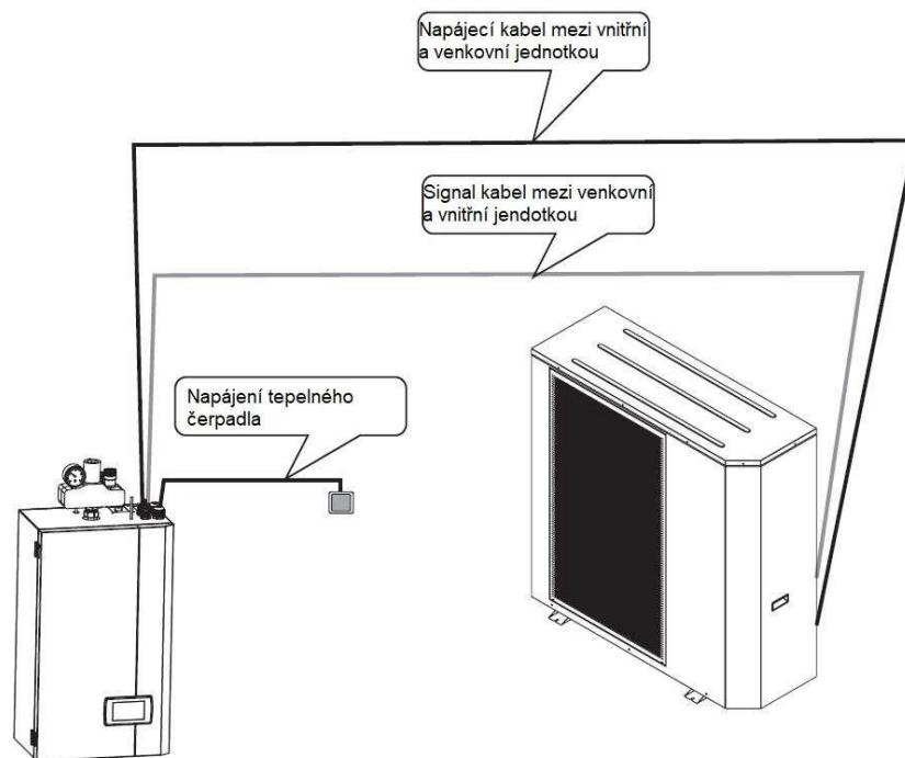
Obr. č. 29 – schéma zapojení
