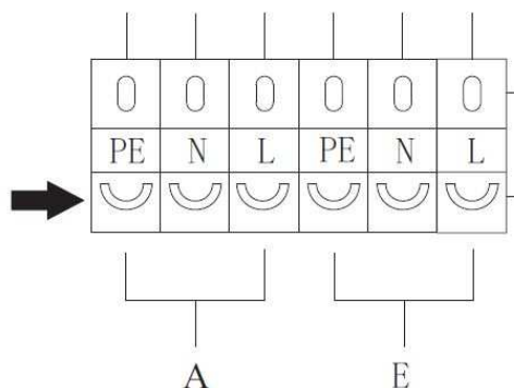
Obr. č. 25 – svorkovnice 1
