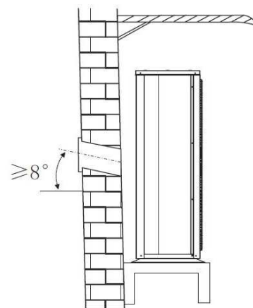
Obr. č. 24 – venkovní jednotka
