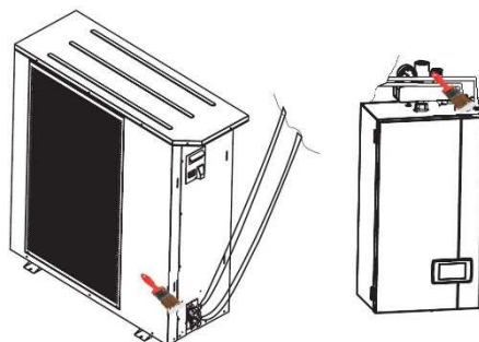
Obr. č. 46 – kontrola těsnosti
